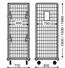
ROLL SÉCURITÉ 4 494 77 03
