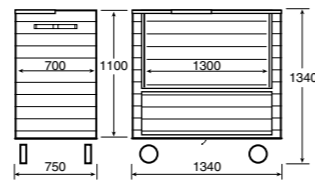
ARMOIRE NAVETTE 2 290 39 11
