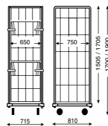
ROLL LINGE 1900 4 494 50 03
