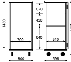
MOBILINGE 2 290 06 11
