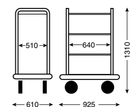
CHARIOT SERVEUR 9 995 30 10
