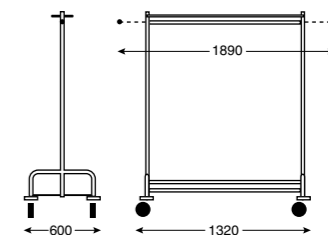
CADDIE PENDERIE 9 972 62 45
