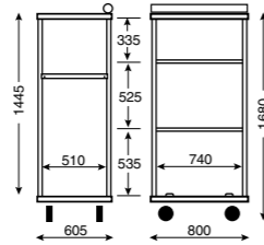
MOBILINGE 2 290 05 11
