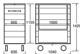
ARMOIRE NAVETTE 2 290 27 11
