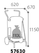
Réf. 57630 avec roues caoutchouc massif
