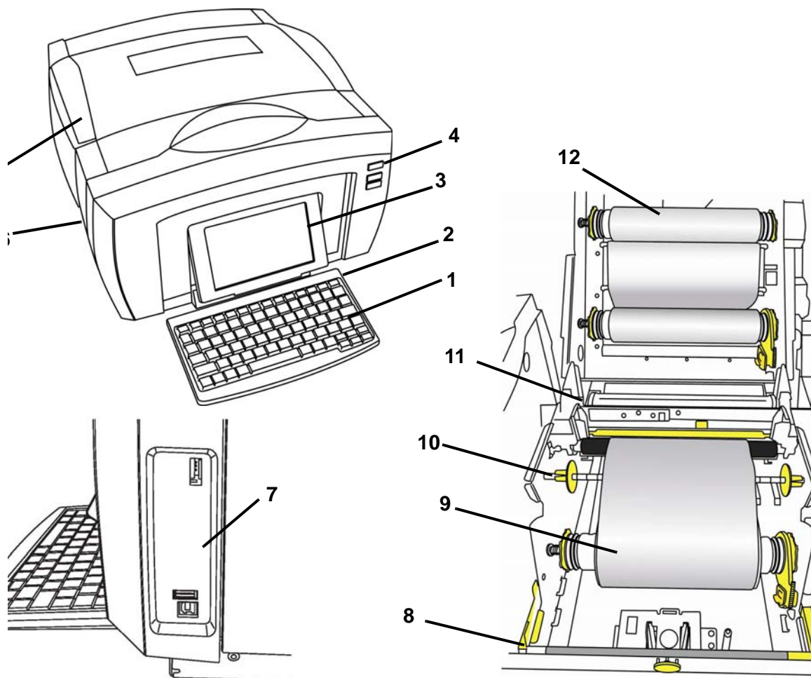
Figure 2-1. Composants de l'imprimante
